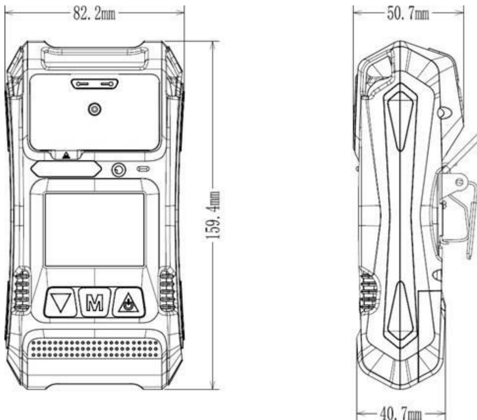
Рис.4: Габаритный чертеж
